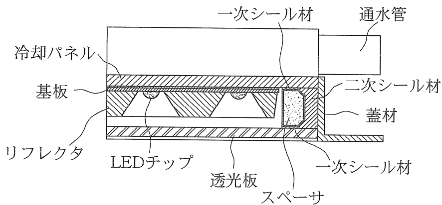
断面図（横）
