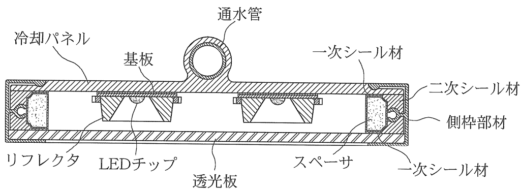
断面図
